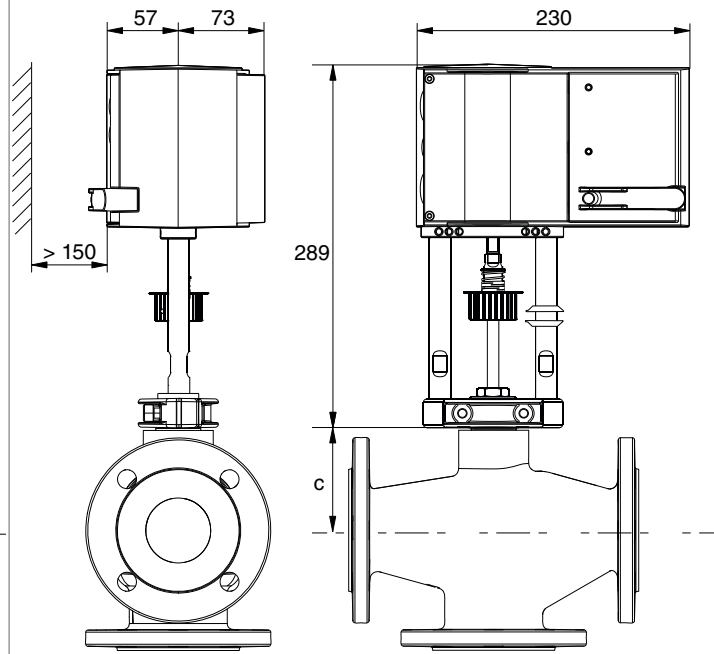
AVF 234
