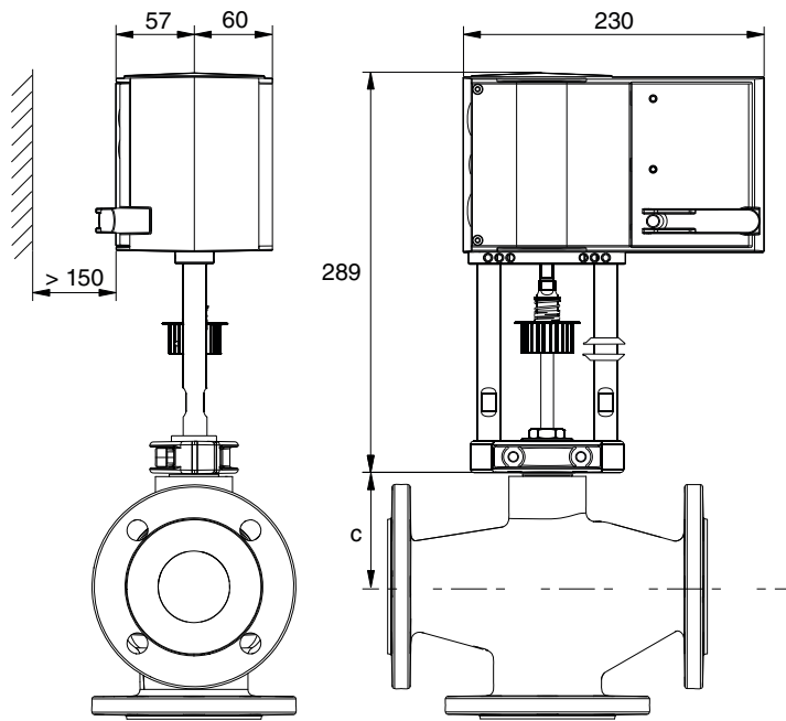
AVM 322(S)
