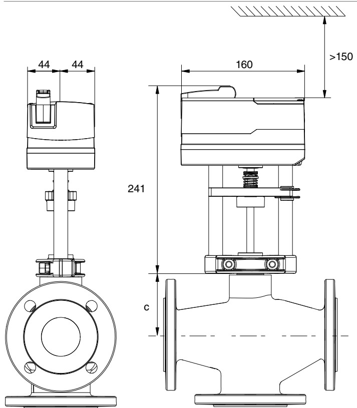
AVM 322(S)
